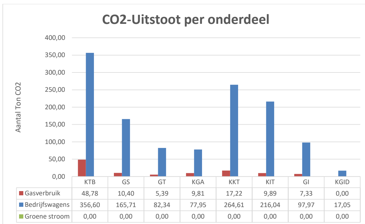
Figuur 5 overzicht uitstoot per bedrijf, per onderdeel
